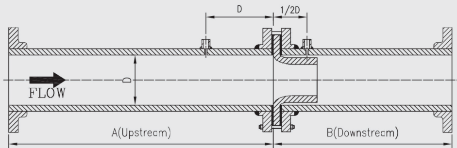
— Flange type —
